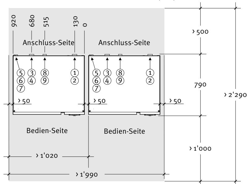
Grundriss (eine oder mehrere Wärmepumpen)
